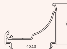
KA-09 آداپتور کنج ۵۰ 460 gr/m rotating frame profiles
