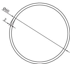
KA-60 لوله محور کنج 980 gr/m axial tube
