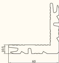
es-501 گونیا ده 2550 gr/m Fixer
