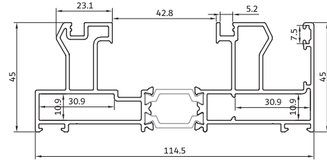
KA-14252.tr چهارچوب کشویی دو ریل 2250 gr/m Rail grid with frame
