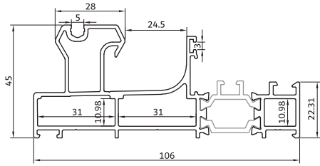
KA-14254.tr چهارچوب کشویی تک ریل 1810 gr/m Rail grid with frame
