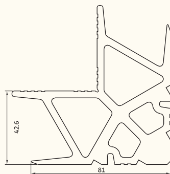
es-504 گونیا ۴۲ 5650 gr/m Fixer
